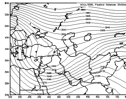
شکل ۱۰. الگوی سینوپتیکی حاکم در تراز ۵۰۰
