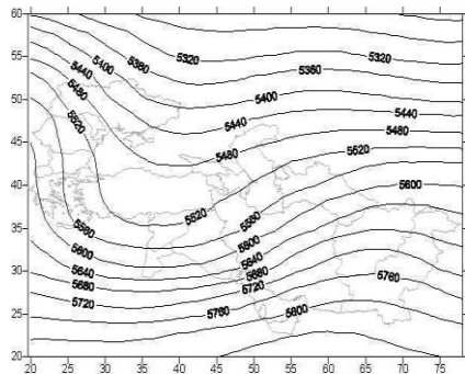
شکل ۸. الگوی سینوپتیکی حاکم در تراز ۵۰۰
