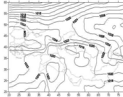
شکل ۹. الگوی سینوپتیکی حاکم در تراز سطح دریا در
