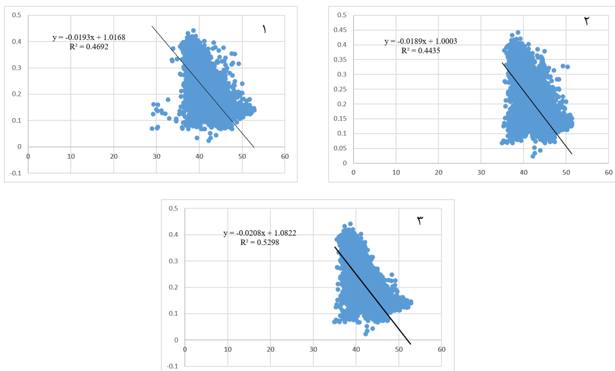
شکل ۷: نمودار همبستگی بین LST و NDVI (۱ سال ۲۰۰۱ تا ۲۰۱۱) سال ۲۰۲۱ (۲ سال ۲۰۱۱ تا ۲۰۲۱) سال ۲۰۲۱
