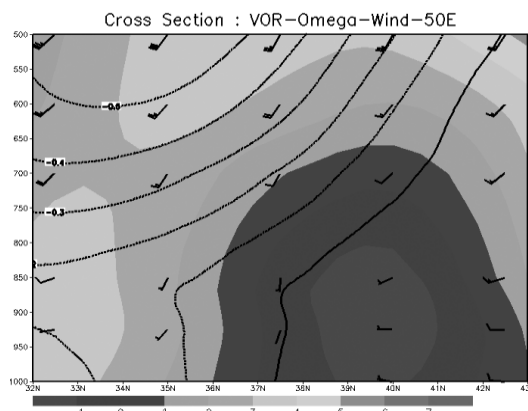
شکل ۲۵: برش قائم میدان تاوایی نسبی (بر ثابته رنگی شده)، برش قائم میدان سرعت قائم (برحسب متر بر ثانیه خطوط هم‌مقدار مشکی رنگ)، برش قائم میدان باد (بر حسب متر بر ثانیه) برای ساعت ۰۹ گرینویچ روز ۱۳ دسامبر ۲۰۱۰.
