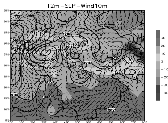
شکل ۴: میدان‌های فشار سطح دریا (خطوط هم‌مقدار بر حسب هکتوپاسکال)، دمای ۲ متری (بخش‌های رنگی شده بر حسب درجه‌ی سلسیوس) و باد ۱۰ متری (بر حسب متر بر ثانیه) برای ساعت ۱۲ گرینویچ روز ۲۹.
