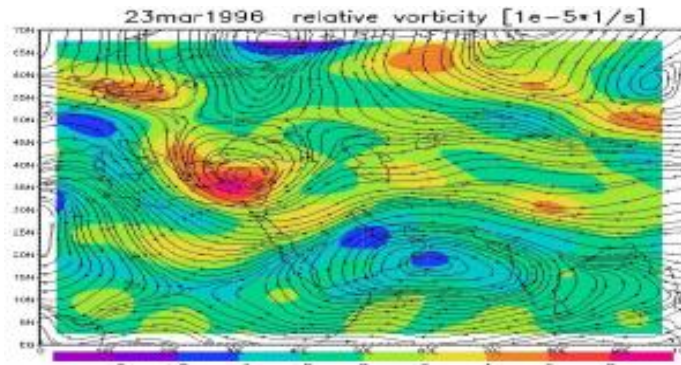
شکل ۶: نقشه تاوایی و خطوط جریان تراز ۱۰۰۰هکتو پاسکال در روز ۲۳ مارس ۱۹۹۶
