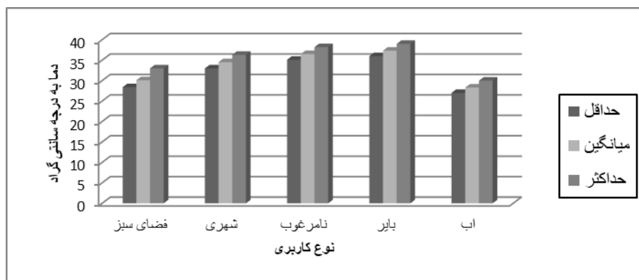
شکل ۵: میانگین دمای سطح زمین برای کاربری‌های مختلف طی سال ۱۹۸۹-۲۰۱۴
