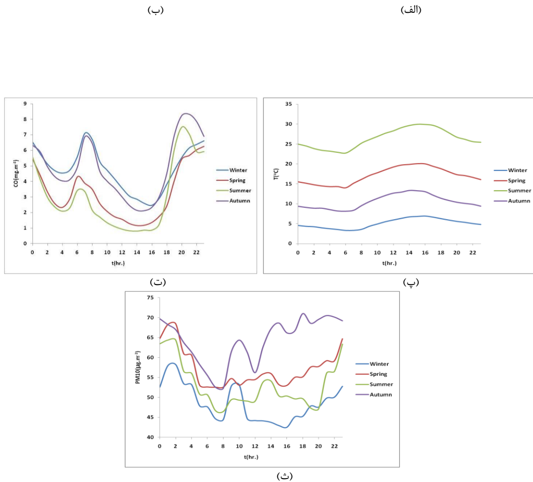
شکل ۸. چرخه‌ی شبانه‌روزی میانگین ساعتی، الف) تندى باد، ب) جهت باد، پ) دما، ت) CO و PM_{10} در فصل‌های مختلف سال ۲۰۰۷.
