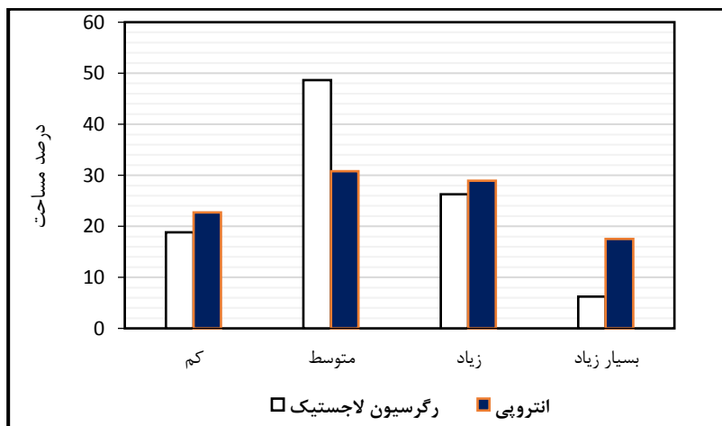
شکل ۶) نمودار توزیع درصد مساحت طبقات ریسک زمین لغزش بر اساس مدل‌های رگرسیون لجستیک و آنتروپیی
