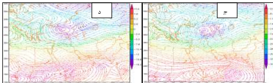
شکل ۶: نقشه‌های وزش دمایی در ترازهای الف: ۱۰۰۰؛ ب: ۸۵۰؛ ج: ۷۰۰۰؛ د: ۵۰۰۰ هکتوپاسکال در روز ۲۹ مارس ۲۰۰۳.
