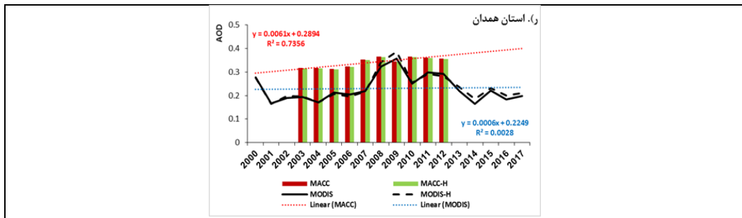
شکل (۳). میانگین سالانه AOD 550nm در استان‌های ایلام، کرمانشاه، کردستان، لرستان و همدان (MODIS & MACC) و ایستگاه‌های سینوپتیک ایلام (I)، کرمانشاه (K)، سنندج (S)، خرم‌آباد (Kh) و همدان (H)
