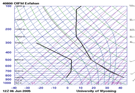
شکل ۳۱. نمودار اسکیتوی ایستگاه اصفهان (الگوی چهارم)
