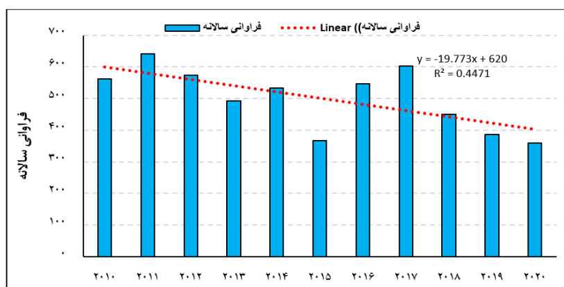
شکل (۳). فراوانی سالانه وارونگی‌های دمایی ایستگاه بندرعباس طی سال‌های ۲۰۱۰ - ۲۰۲۰
