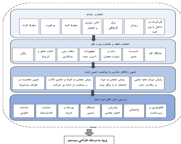
شکل ۱: مدل مفهومی کاربردی اینترنت اشیا برای کاهش حوادث و ارتقای ایمنی فضاهای کارگاهی ساختمانی تهران
