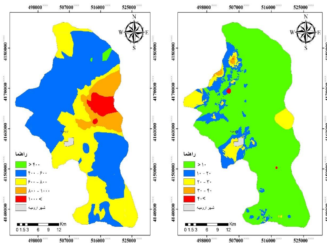
شکل ۶. میزان برداشت از چاه‌های آب زیرزمینی
