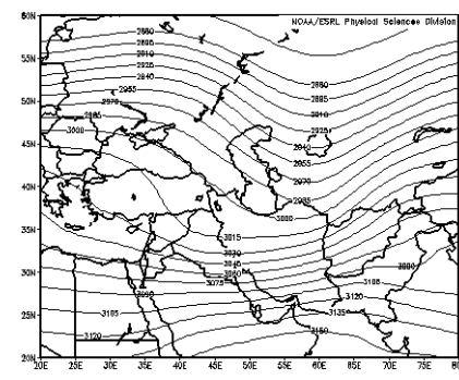
شکل ۱۶. الگوی سینوپتیکی حاکم در تراز ۷۰۰ هکتوپاسکال در روز همراه با بارش برف (الگوی CP۴)
