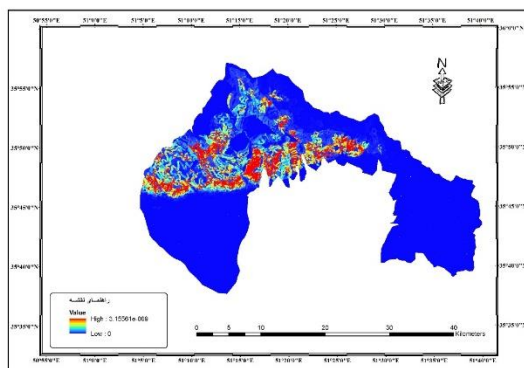
شکل ۲۲. پهنه‌بندی خطر زمین‌لغزش با عملکرد ضرب فازی.
