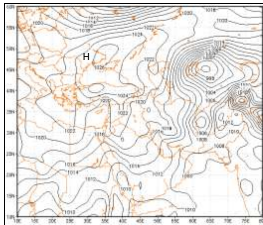
شکل ۱۰: نقشه‌ی فشار تراز دریا روز ۲۵ مارس ۲۰۰۵.
