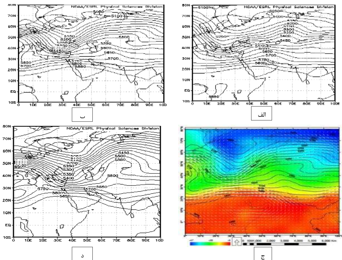
شکل ۲: نقشه‌ی الگوی فشار سطح ۵۰۰ هکتوپاسکال. الف) روز ۱۷ ژانویه ۱۹۸۶ (روز قبل از وقوع کولاک)؛ ب) روز ۱۸ ژانویه ۱۹۸۶ (روز رخداد کولاک)؛ ج) نقشه‌ی ترکیبی فشار سطح ۵۰۰ با دما و باد روز ۱۸ ژانویه ۱۹۸۶ (روز رخداد کولاک)؛ د) روز ۱۹ ژانویه ۱۹۸۶ (روز بعد از رخداد کولاک).
