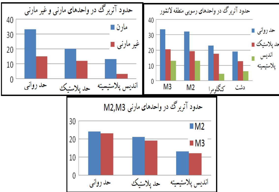
شکل ۵: میانگین حد روانی، حد خمیری و شاخص خمیری در کل واحدهای کاری (بالاراست)، در واحدهای مارنی و غیرمارنی (بالاچپ) در دو واحد مارنی حوزه آبخیز لانتشور (پایین)
