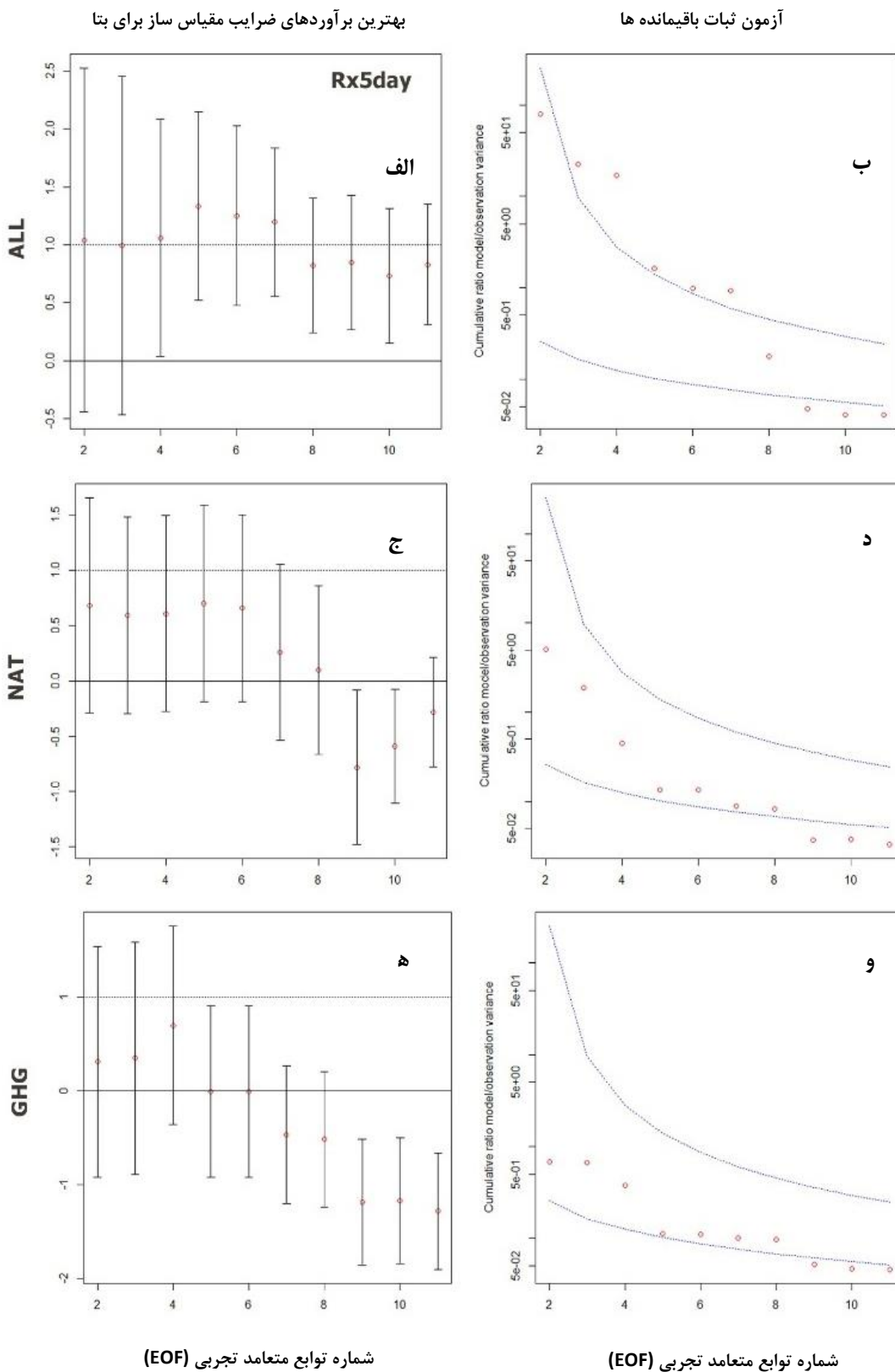
شکل ۲: بهترین ضرایب مقیاس ساز برای سیگنال های ALL, NAT, GHG مربوط به Rx5day (کادر سمت چپ) و نتایج آزمون ثبات باقیمانده ها (کادر سمت راست)
