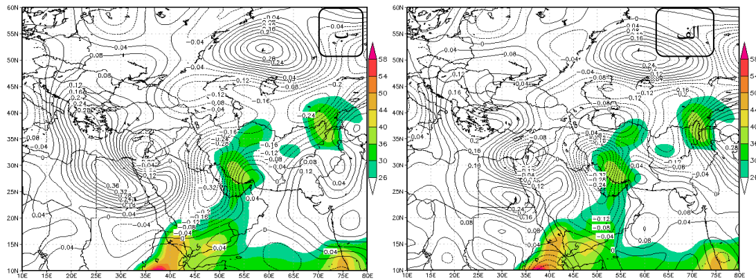
شکل ۷. نقشه‌های ترکیبی مجموع رطوبت (۱۰۰۰-۵۰۰) و امگا برحسب پاسکال بر ثانیه در ترازهای الف: ۷۰۰، ب: ۵۰۰
