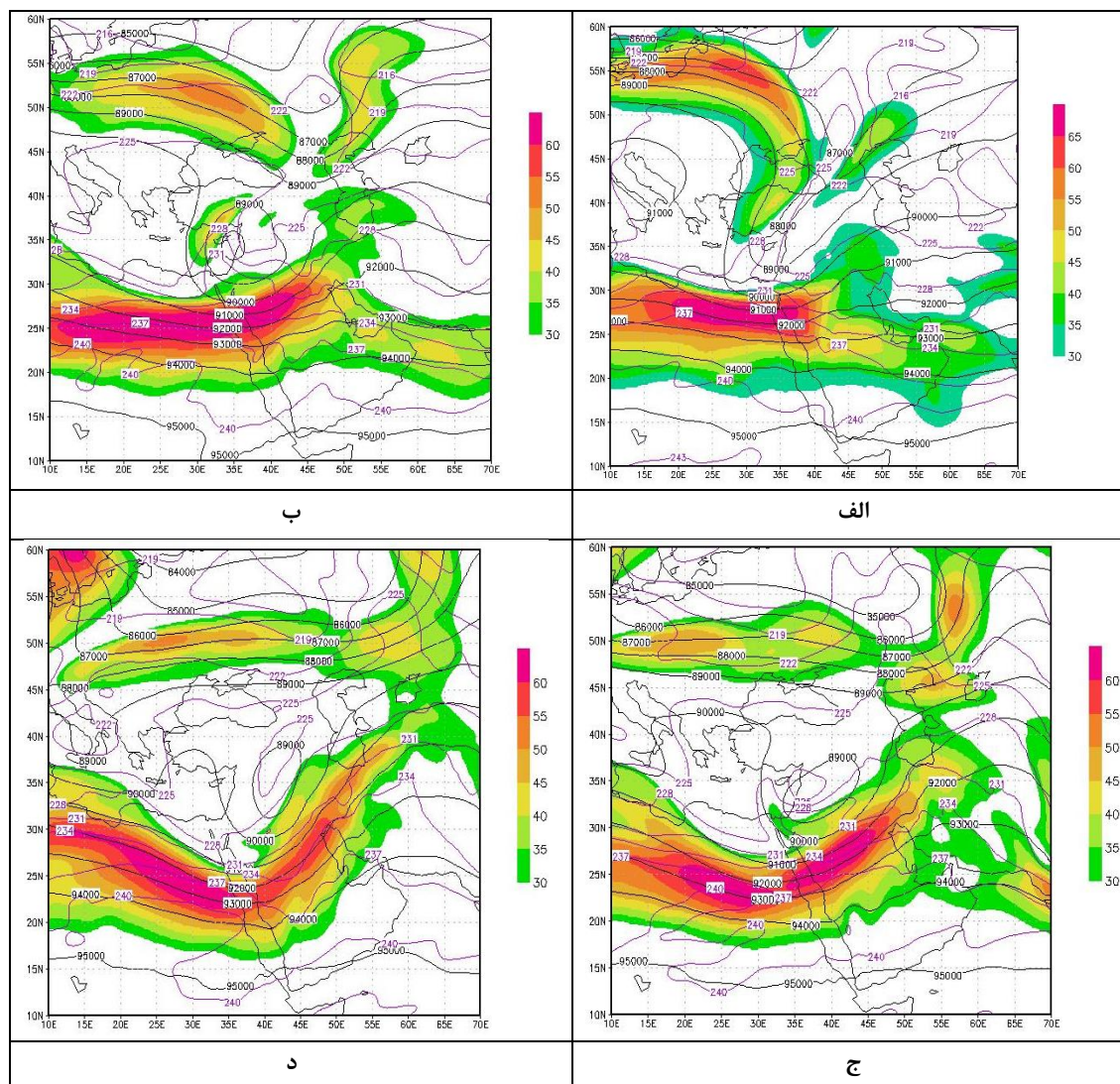
شکل ۵. نقشه‌ی ارتفاع ژئوپتانسیل (خطوط سیاه)، دما (خطوط بنفش) و سرعت باد (سطوح رنگی) سطح ۳۰۰ ه. پ. در الف)
