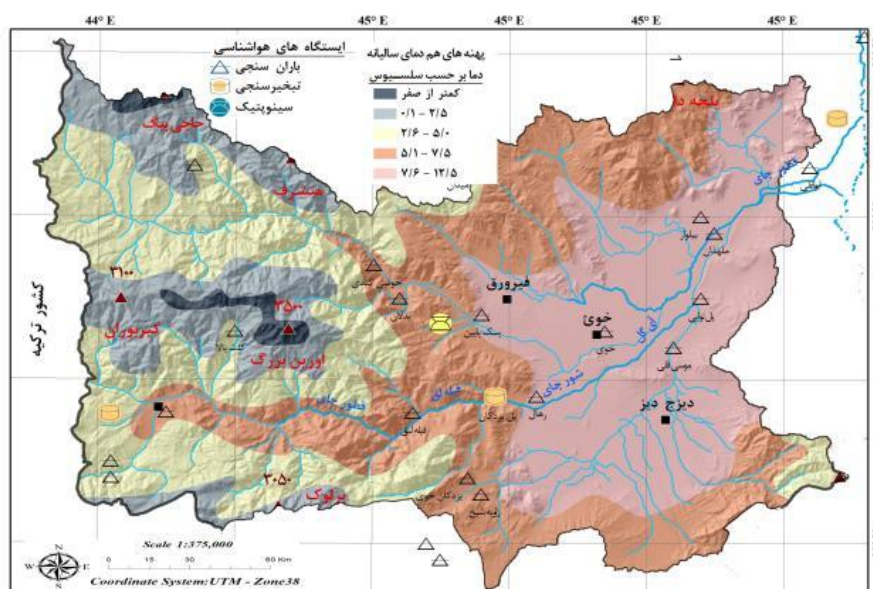
شکل ۲. پهنه‌های هم‌دمای سالانه حوضه آبخیز قطورچای
