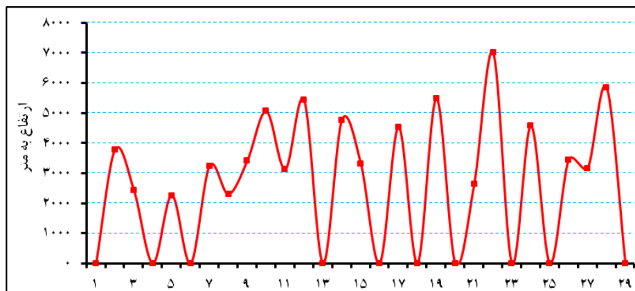
شکل ۸. تغییرات روزانه عمق لایه آمیخته در ساعت ۱۲ UTC در ماه فوریه ۲۰۱۲: (روزهایی که عمق لایه صفر نشان داده شده است هیچ نوع وارونگی ای مشاهده نشده است).
