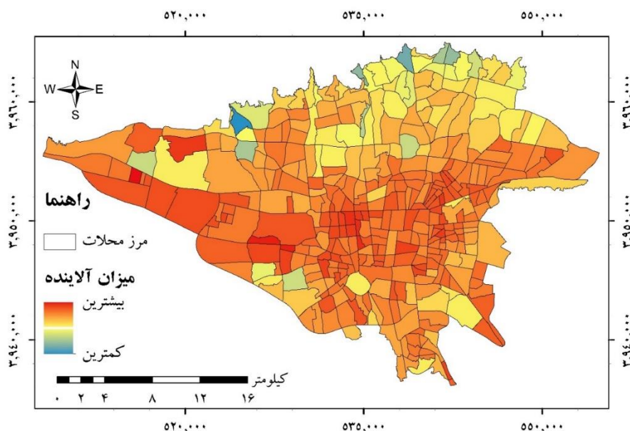
شکل ۵. نقشه تغییرات فضایی PM_{10} شهر تهران
