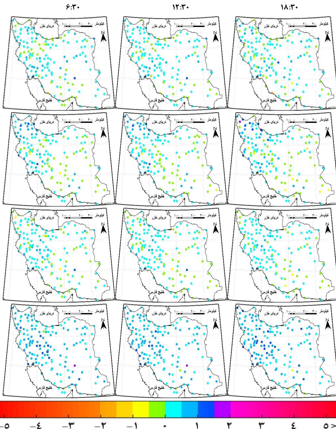
شکل ۴ پراکندگی فصلی روند (به ازای هر ده سال) برای دمای عمق ۲۰ سانتی‌متری خاک در ساعت‌های ۹:۳۰ صبح، ۱۲:۳۰ ظهر و ۱۸:۳۰ عصر در ایران (از بالا به پایین بهار تا زمستان)
