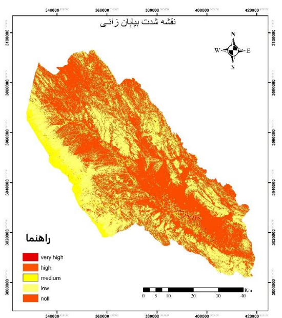
شکل (۵). نقشه شدت بیابان‌زایی حاصل از معادله I = a * \text{NDVI} - \text{Albedo}
