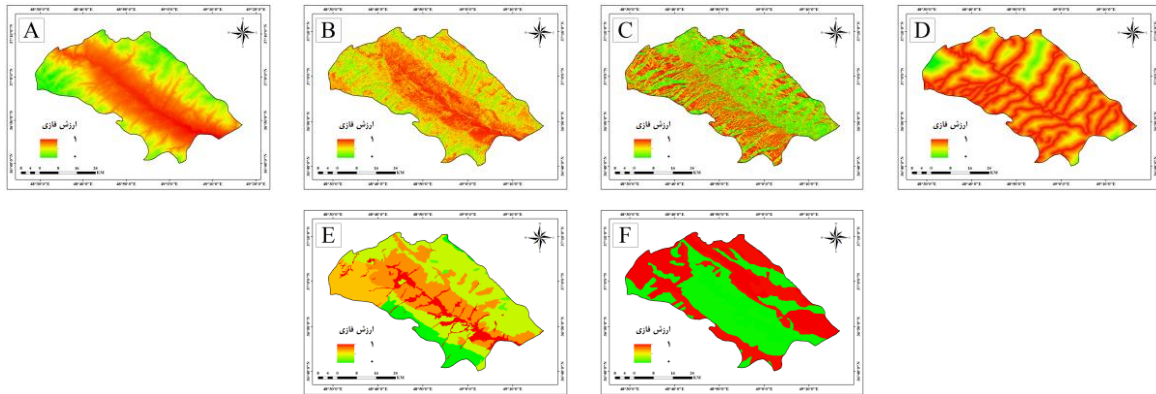
شکل ۳. فازی سازی لایه‌های اطلاعاتی جهت شناسایی مناطق مستعد وقوع سیلاب
